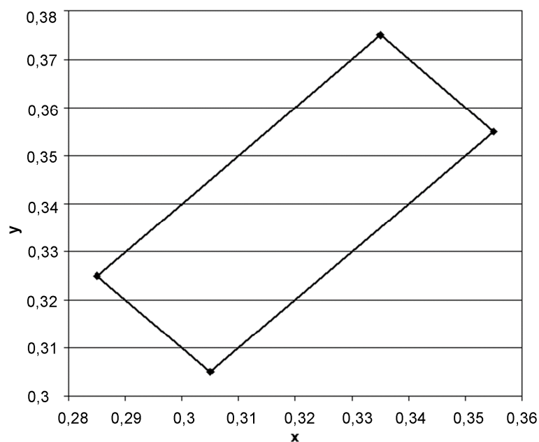
Rys. 1. Współzrędnymi chromatyczności x,y dla barwy białej oznakowania
