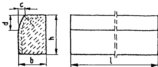
rys. 1 Wymiary krawężników
